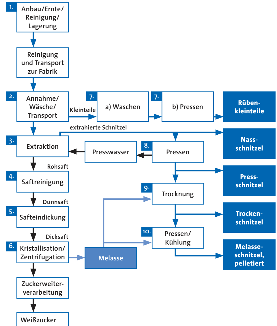
Abbildung 1: Prozessschema
